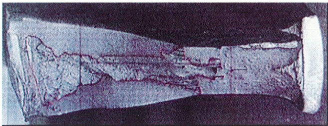
c) 第Ⅲ类异常断口
