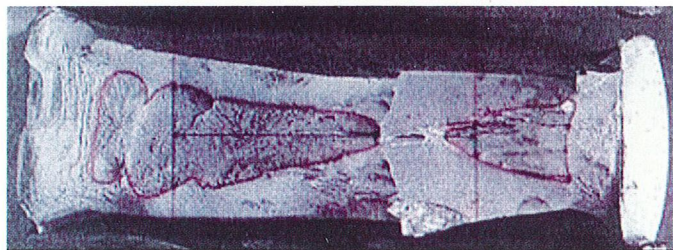
d) 第Ⅳ类异常断口
